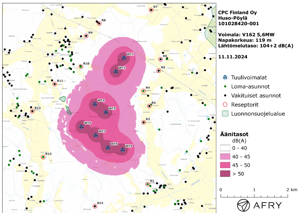
Kuva 3-2: Keskiäänitasot LAeq Huso-Pöylän tuulivoimapaiston hankealueella.
