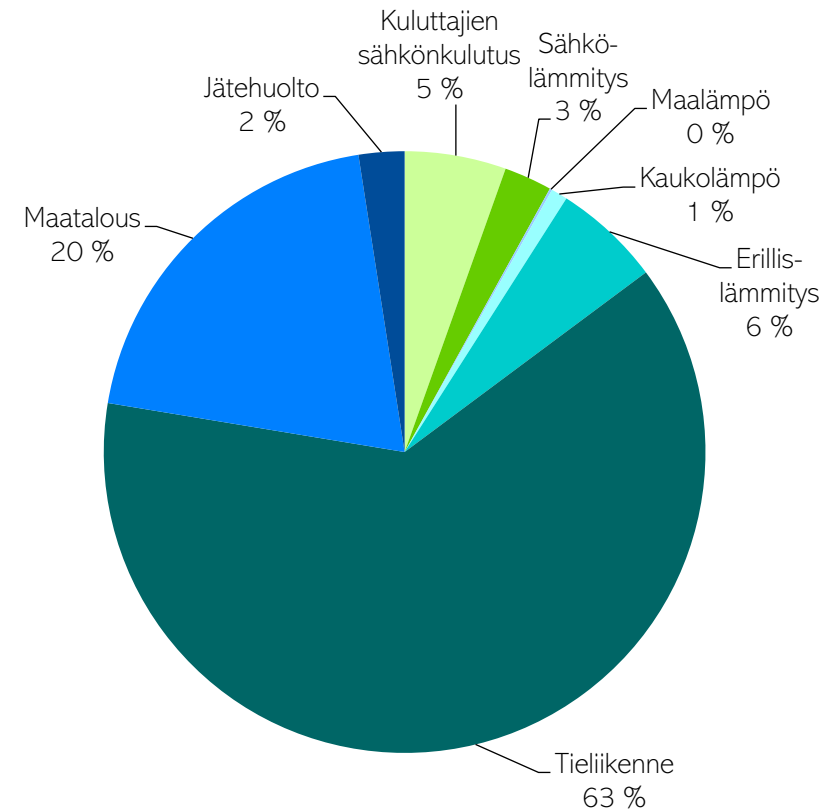
Kuva 1. Paimion päästöt sektoreittain vuonna 2023 ilman teollisuutta. (CO 2 -raportti, 2025)
