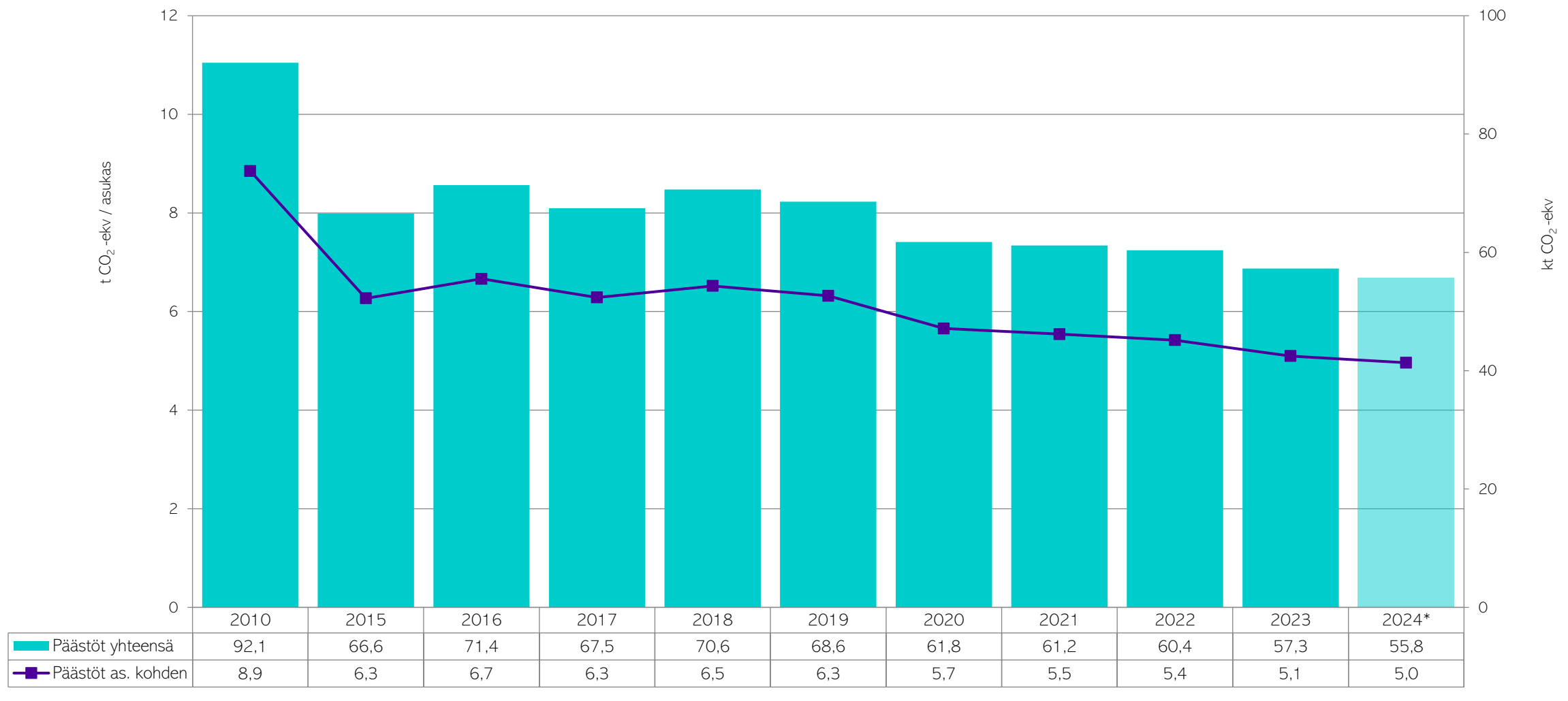
Kuva 3. Päästöt yhteensä ja asukasta kohden Paimiossa vuonna 2010 ja vuosina 2015–2024 ilman teollisuutta. Vuoden 2024 tieto on ennakkotieto. (CO2-raportti, 2025)
