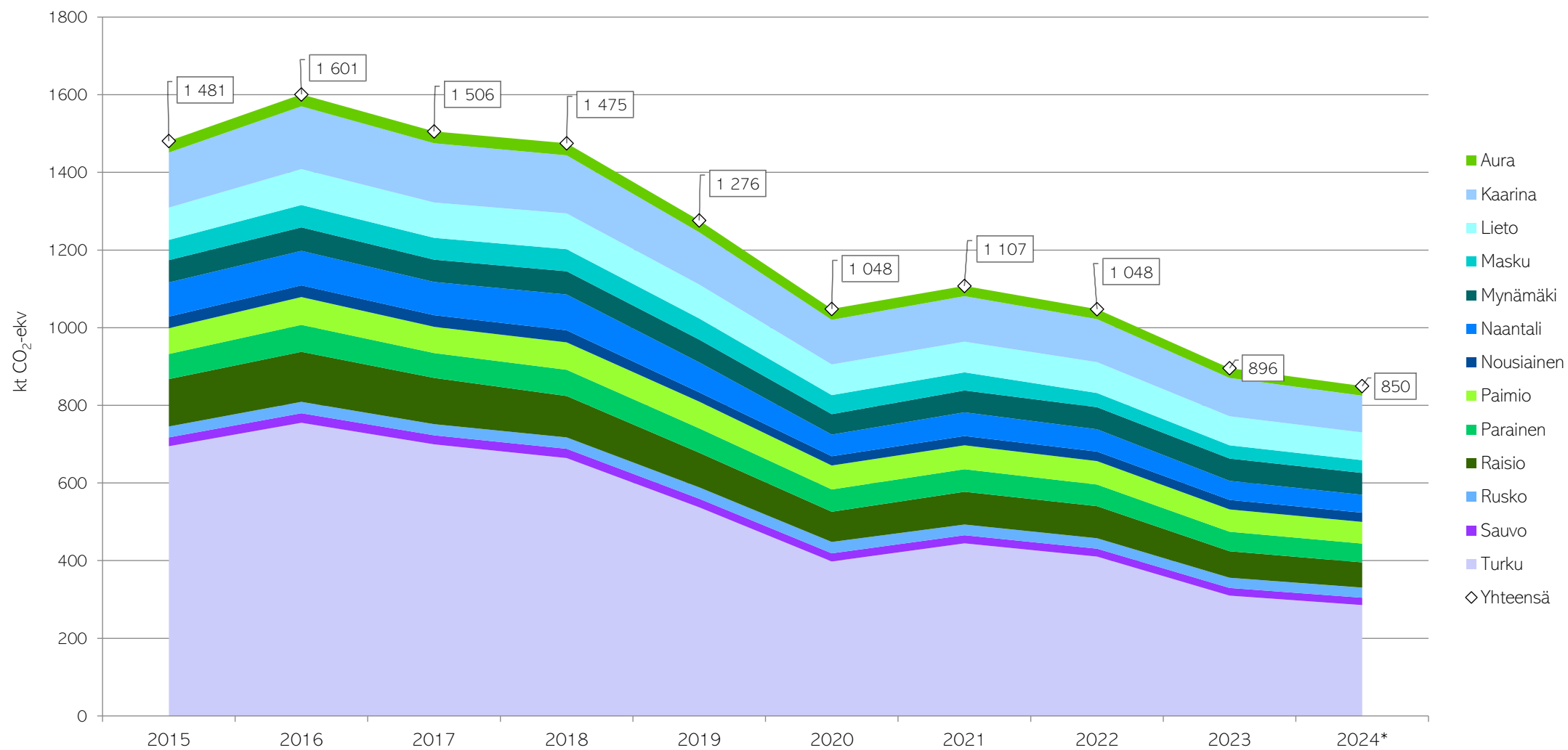
Kuva 13. Turun kaupunkiseudun kuntien kasvihuonekaasupäästöt yhteensä vuosina 2015–2024. Vuoden 2024 tieto on ennakkotieto. Teollisuuden päästöt eivät ole mukana tarkastelussa. Kasvihuonekaasupäästöt ovat TKS-kuntien yksi MAL-sopimuksen vaikuttavuuden indikaattori. ( CO 2 -raportti , 2025)
