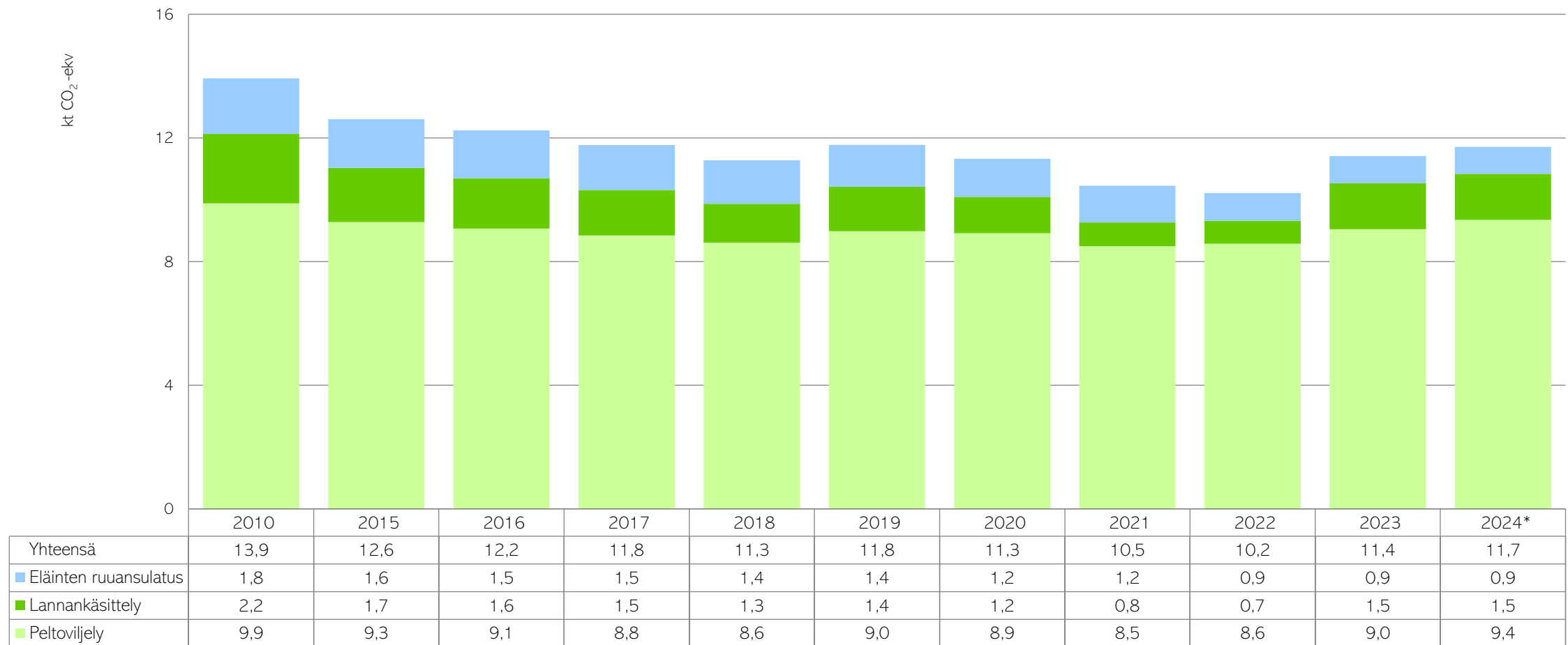
Kuva 7. Maatalouden päästöjen kehitys Paimiossa vuonna 2010 ja vuosina 2015–2024 jaettuna eläinten ruuansulatuksen, lannankäsittelyn ja peltoviljelyn päästöihin. Vuoden 2024 tieto perustuu osittain ennakkotietoihin. (CO 2 -raportti, 2025)
