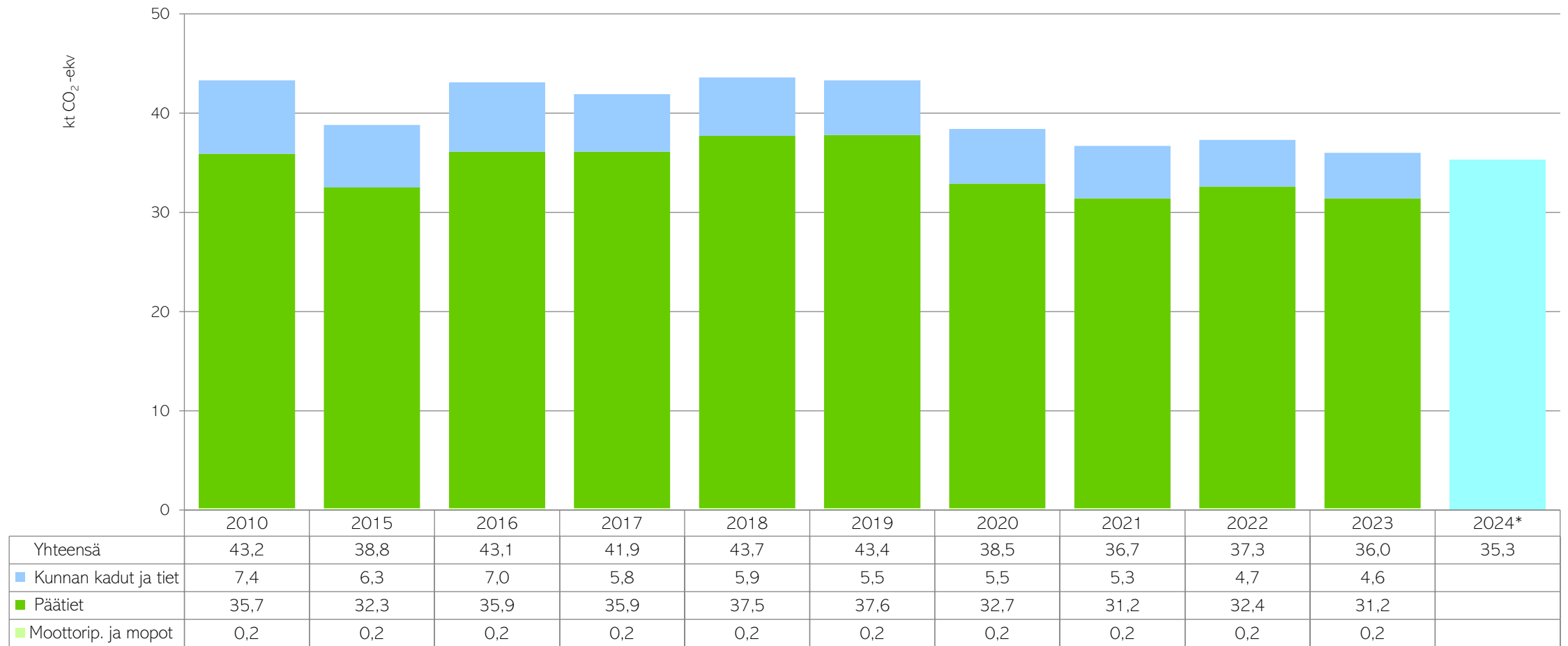
Kuva 6. Tieliikenteen päästöt Paimiossa vuonna 2010 ja vuosina 2015–2024. Vuoden 2024 tieto on ennakkotieto. (CO 2 -raportti, 2025)
