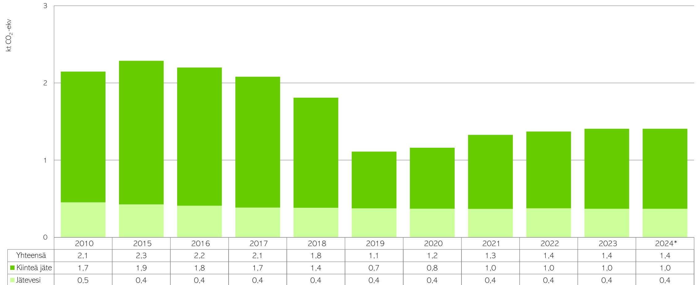
Kuva 8. Jätehuollon päästöjen kehitys Paimiossa vuonna 2010 ja vuosina 2015–2024. Vuoden 2024 ennakkotietona on vuoden 2023 tieto. (CO 2 -raportti, 2025)
